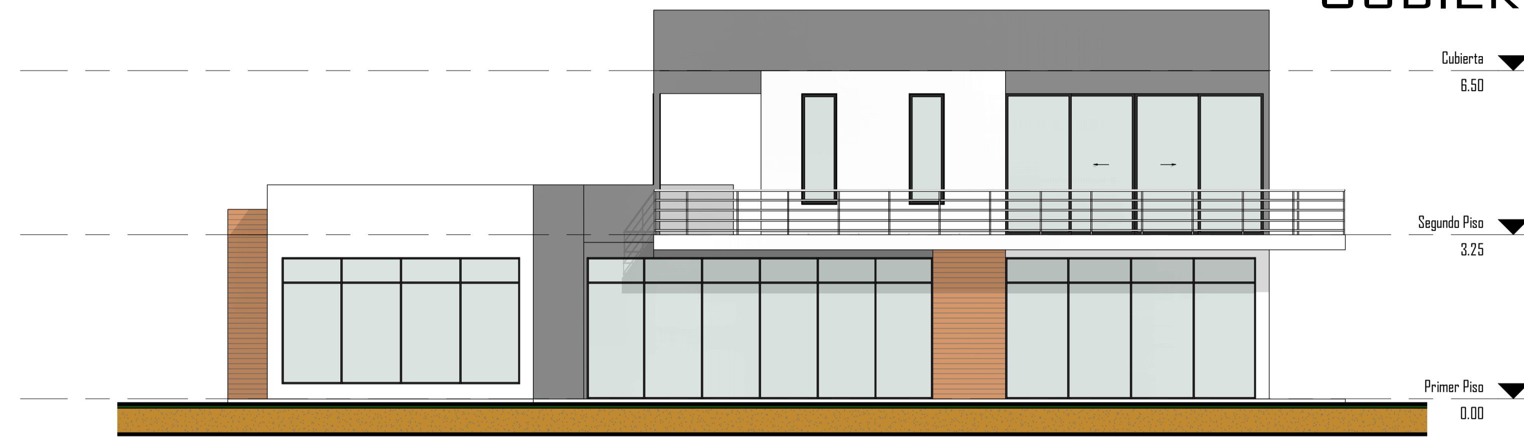
4 Fachada Lateral Derecha 1:75
