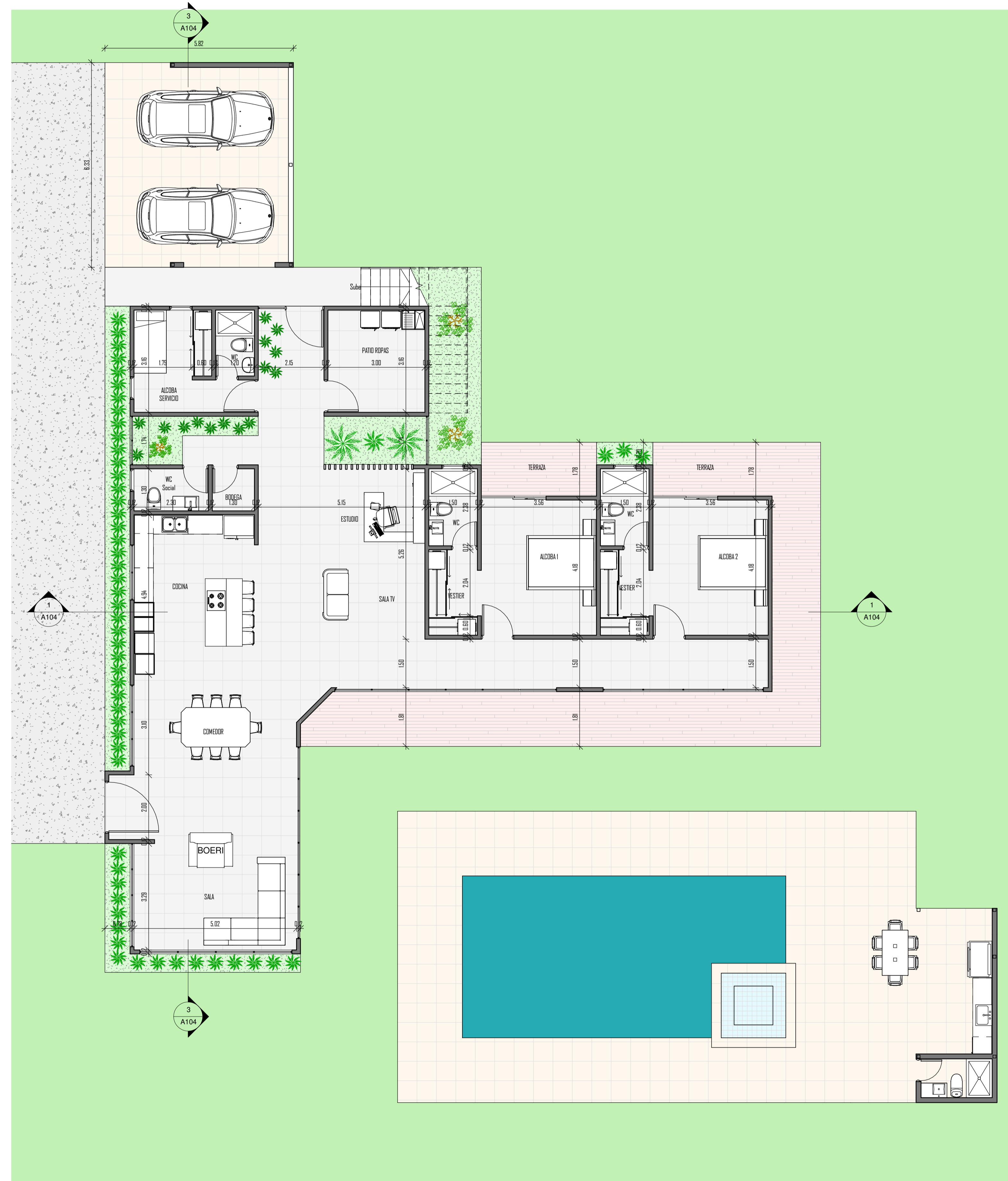
1 Primer Piso 1:75
