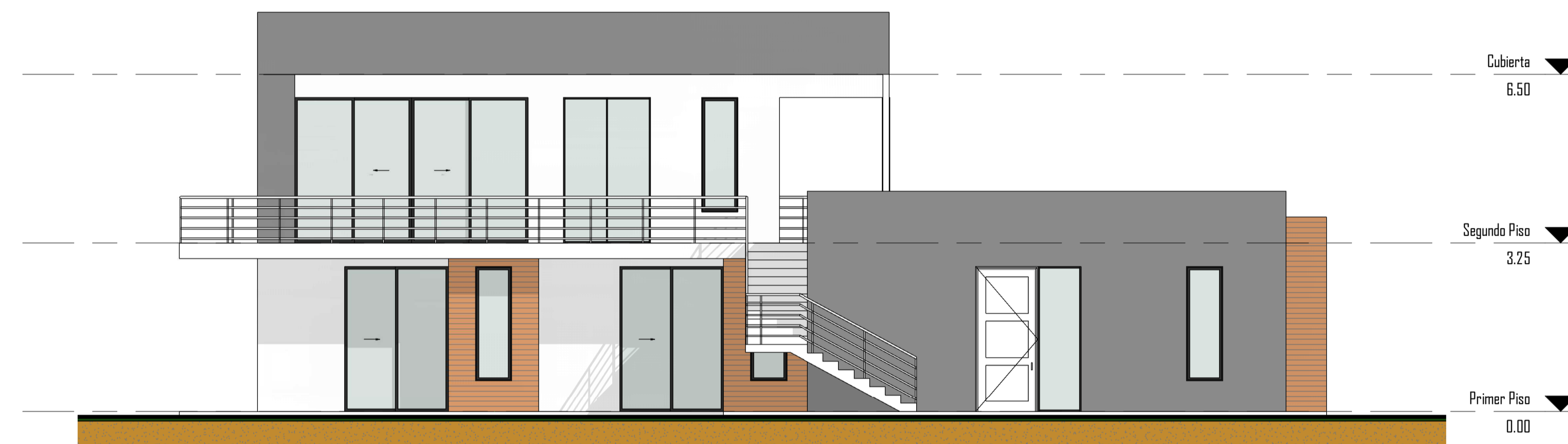
5 Fachada Lateral Izquierda 1:75
