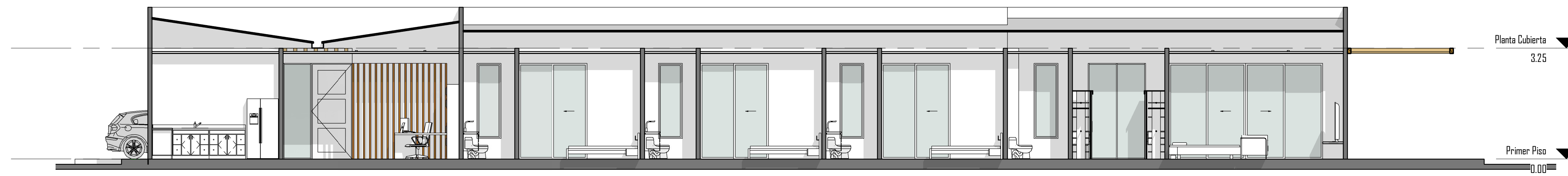
1 Sección 1 1:75
