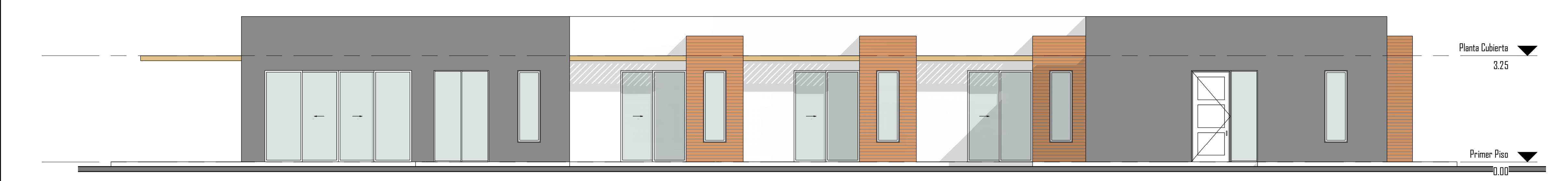
4 Fachada Lateral Izquierda 1:75
